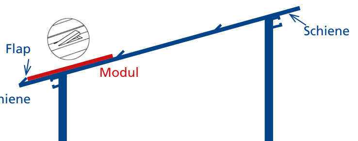
Die Flaps verhindern das Zurückrutschen und halten die Module in der korrekten Position.
